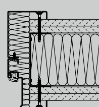
Rohová a přidavná zárubeň Montáž pomocí šroubů
